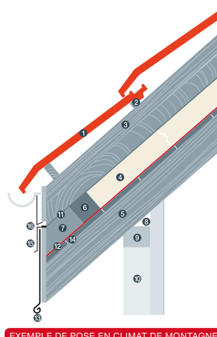
EXEMPLE DE POSE EN CLIMAT DE MONTAGNE
