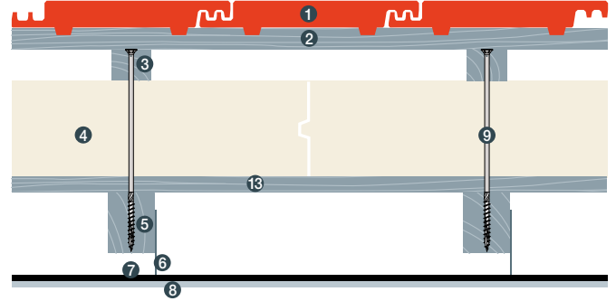
> POSE SUR PLATELAGE BOIS
