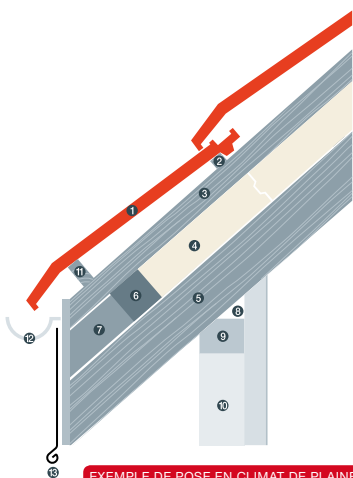
EXEMPLE DE POSE EN CLIMAT DE PLAINE
