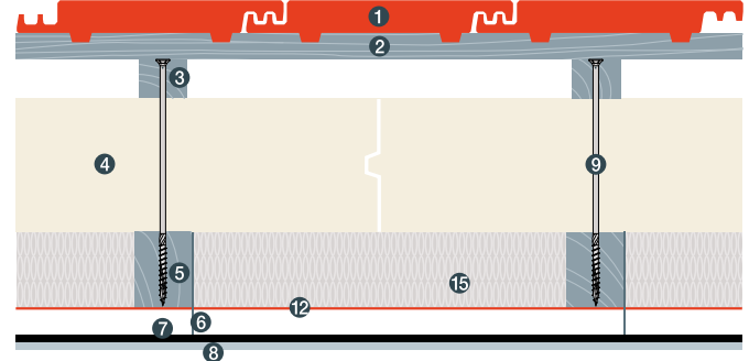
> POSE SUR CHEVRONS AVEC UNE ISOLATION EXISTANTE
